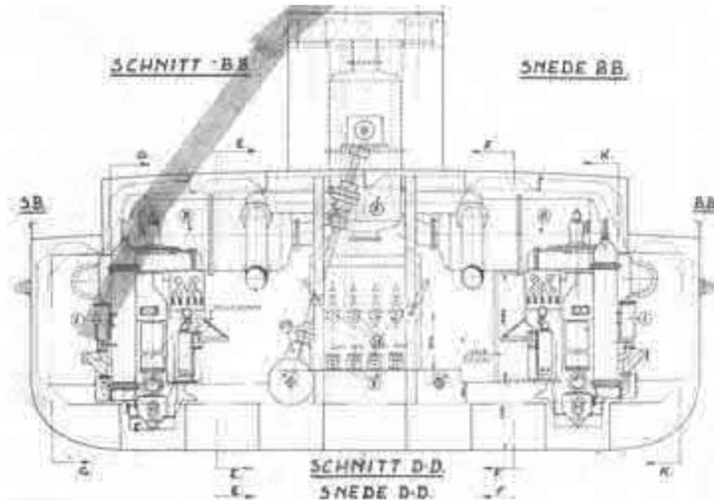
Stranglierenantrieb (Schleppwindenantrieb)
